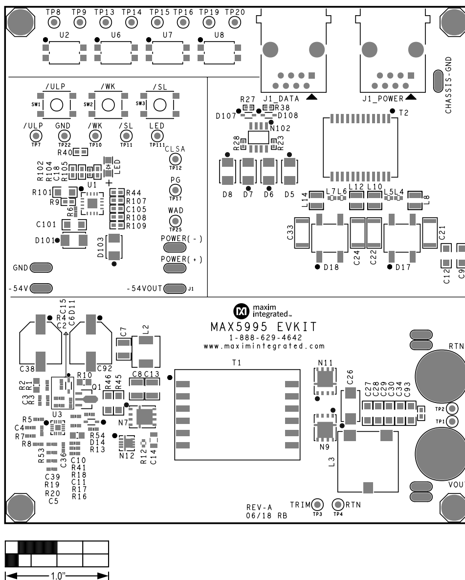
MAX5995 EV—Top Silkscreen
