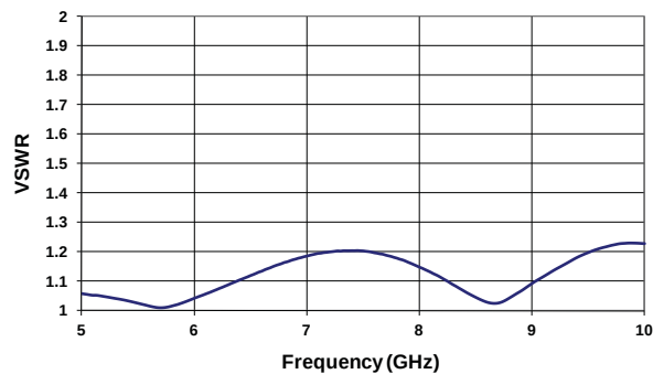
VSWR (5-10 GHz)
