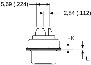
DD Configuration
