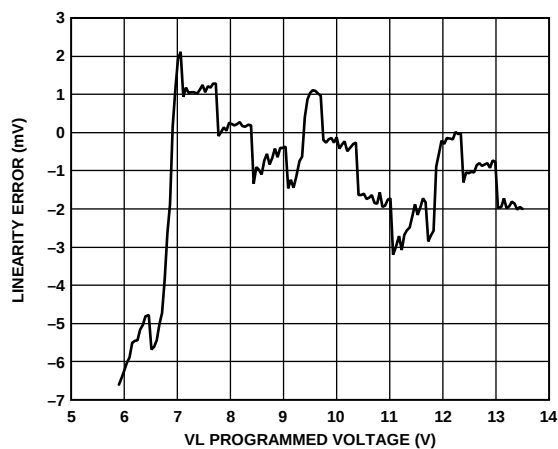
Figure 27. HVOUT VHH Linearity Error
