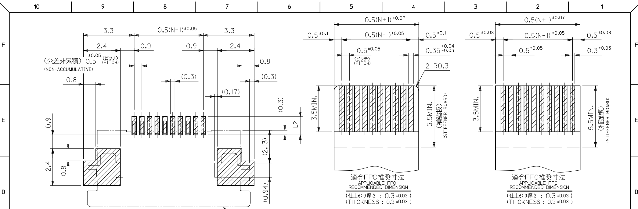
コネクタ位置 CONNECTOR POSITION
