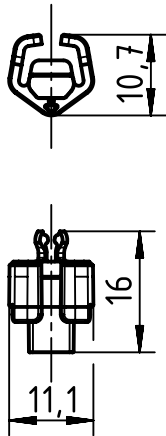
Coding Pin
