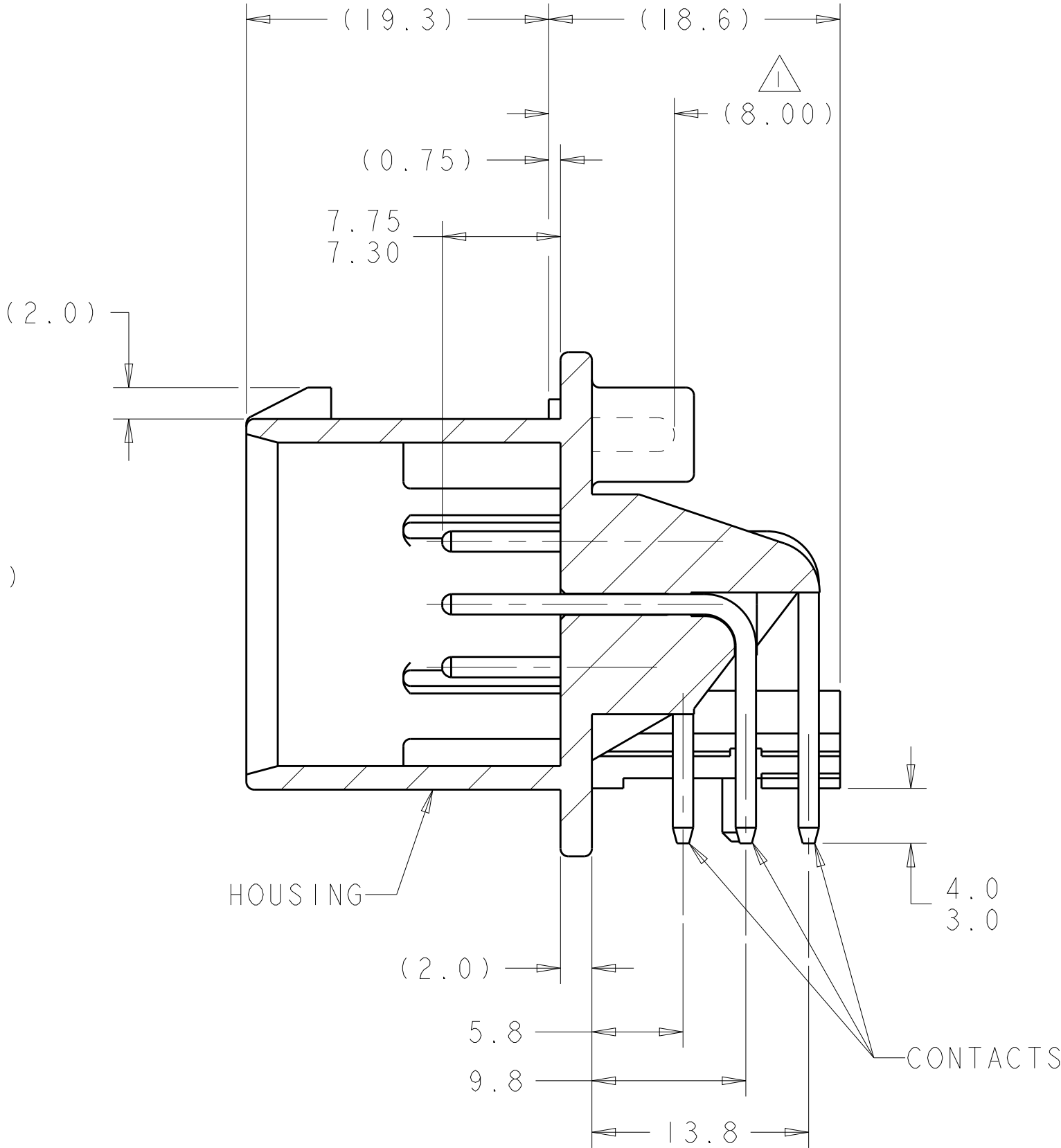
SECTION A-A
