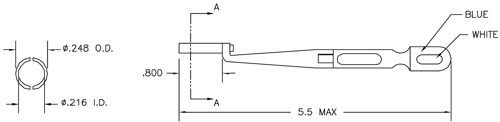
VIEW A-A
