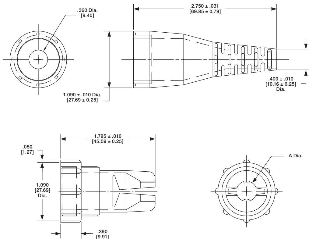
Cable Grip
