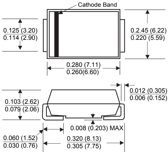
DO-214AB (SMC J-Bend)
