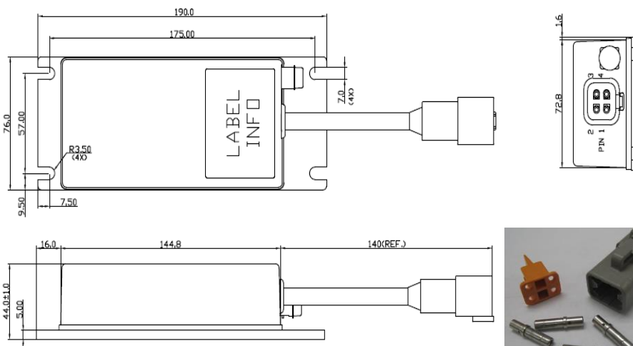
B62SR13722BC
