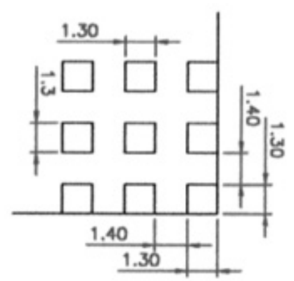
A-A SCALE 4:1
