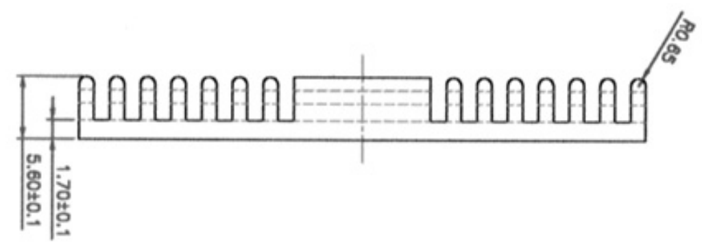
A-A SCALE 4:1
