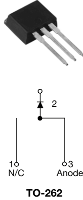
VS-30ETH06-1PbF
