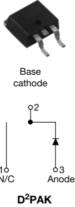
VS-30ETH06SPbF
