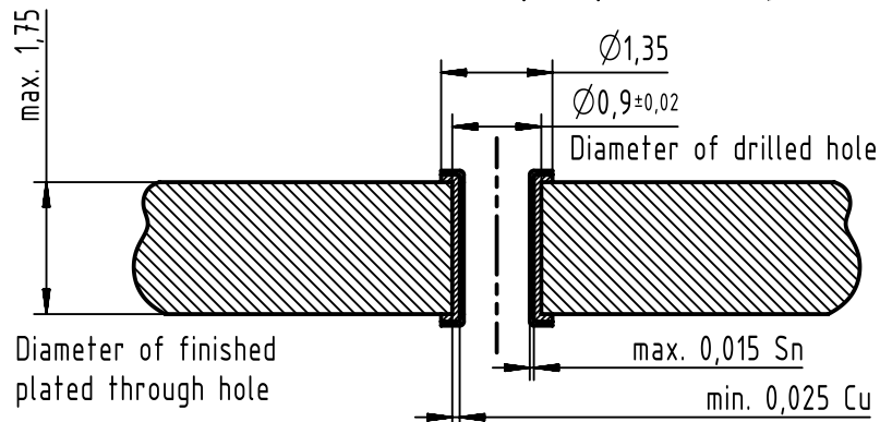
A-A (10:1)
