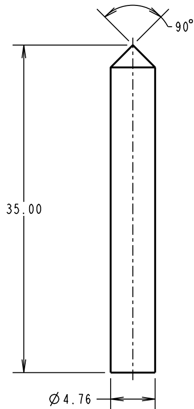
Z10002-00 TOP TOOL
