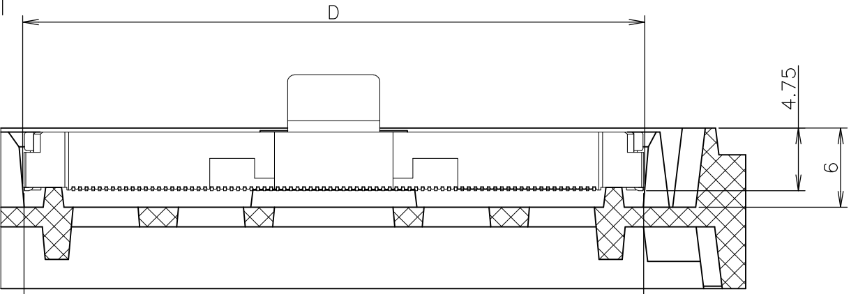
SECT.A-A
