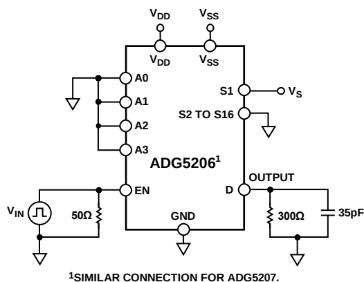
Figure 36. Enable Delay, t_{ON}(EN) , t_{OFF}(EN)
