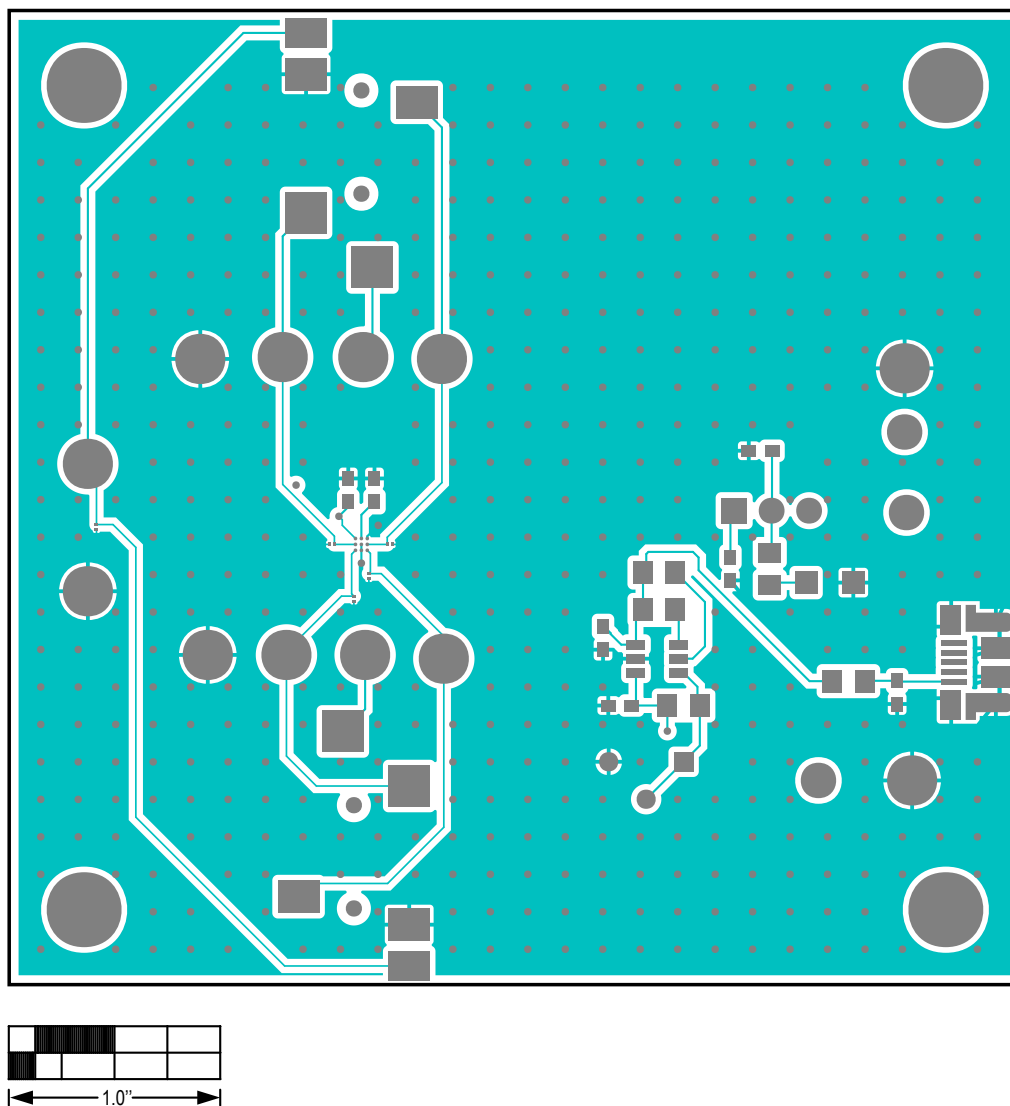
MAX20331 EV Kit—Top Layer
