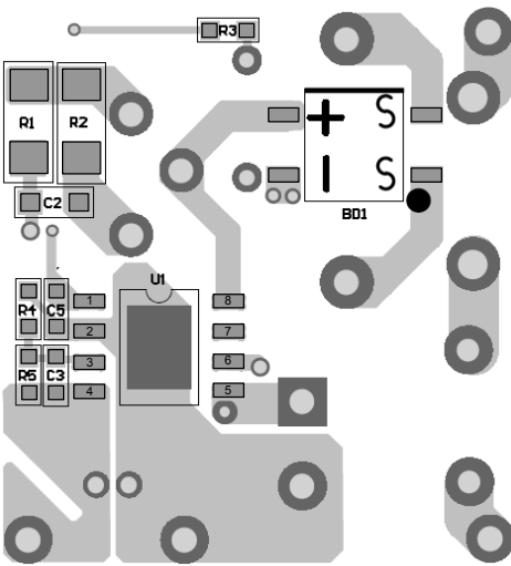
Bottom Layer
