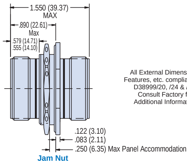
Jam Nut
