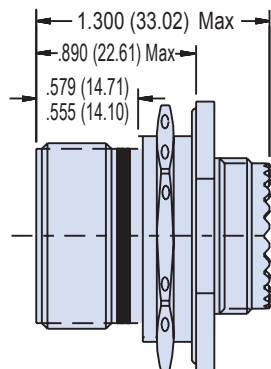
Jam Nut
