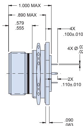
Jam Nut Receptacle
