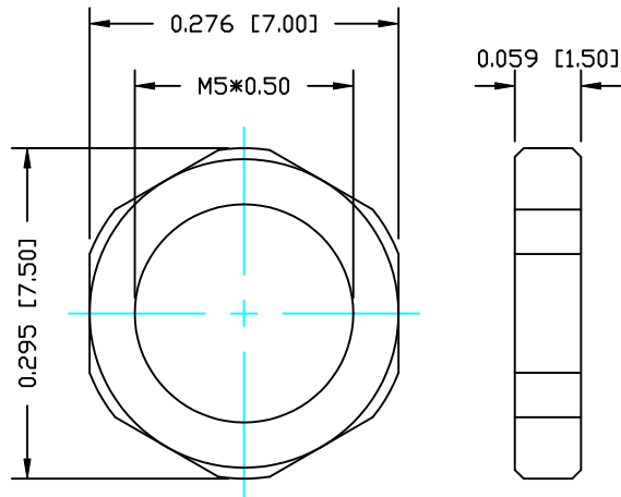
NUT
