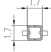
SEC D-D
