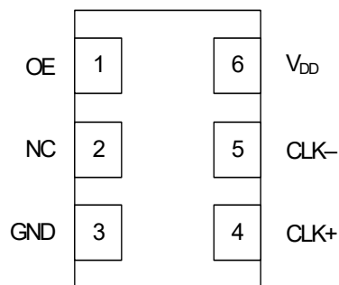
Si531 LVDS/LVPECL/CML
