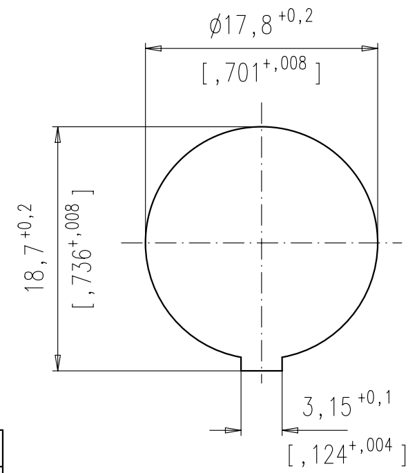
Montageausschnitt Panel Cutout
