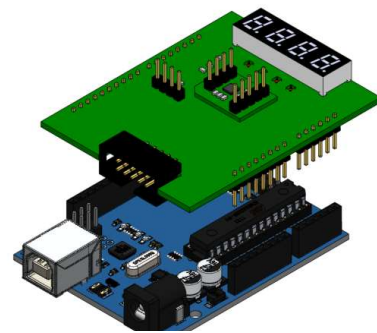
IQS621 Shield + Arduino Uno 1
