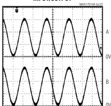
A: INPUT SIGNAL, 5V/div B: OUTPUT SIGNAL, 5V/div
