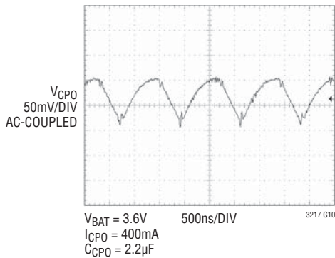
1.5x Mode CPO Output Ripple
