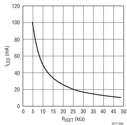
I_{\text{LED}} vs R_{\text{SET}}
