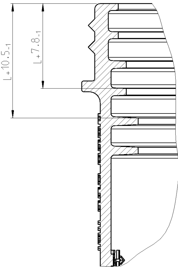
SECTION A-A Schnitt SCALE 5:1 Maßstab
