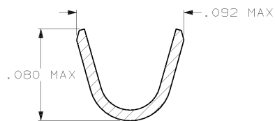
SECTION A-A SCALE 20:1
