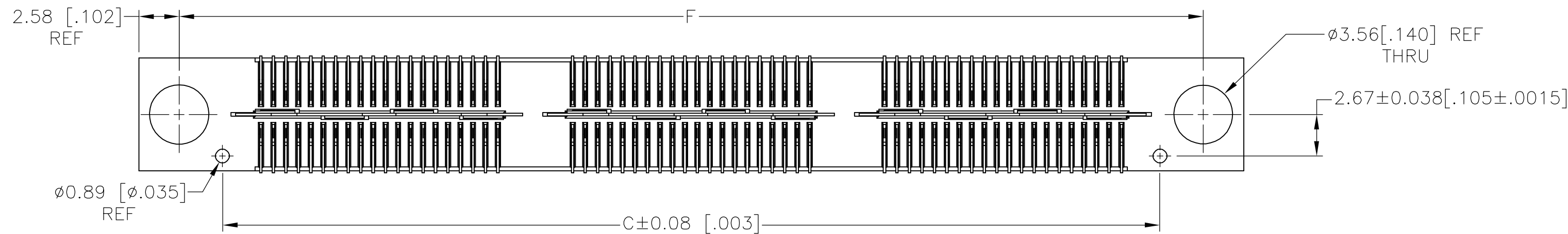
SECTION A-A
