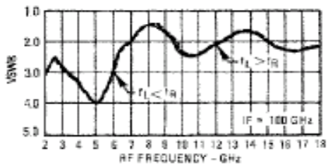
R-Port VSWR
