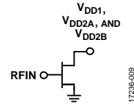
Figure 9. V DD1 , V DD2A and V DD2B Interface Schematic
