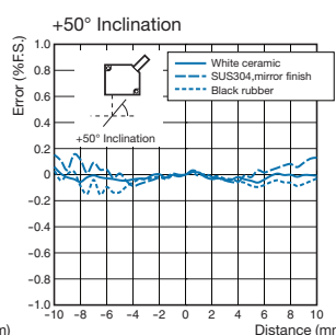
+50° Inclination
