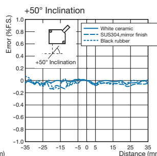
+50° Inclination
