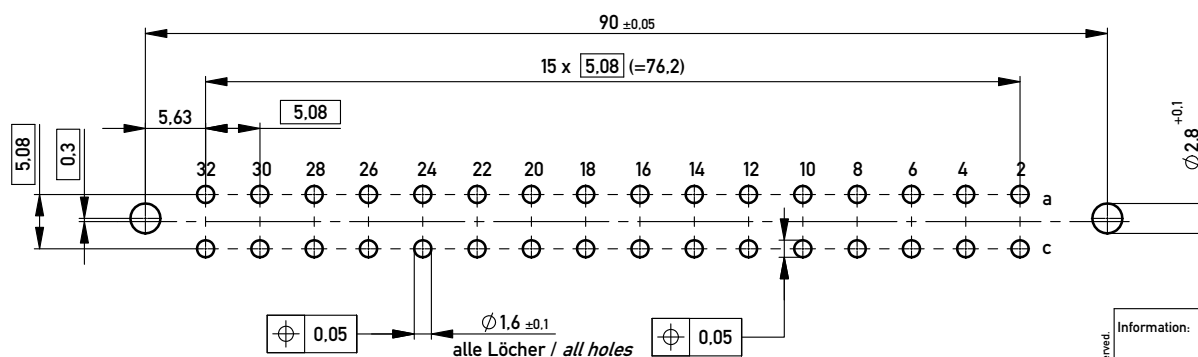
Leiterplatten-Layout Vorschlag PCB-Layout proposal
