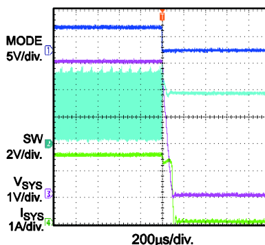
Mode Off, Boost Mode V_{SYS\_SET}=5V , V_{BATT}=3.7V , R_{SYS\_LOAD}=2\Omega
