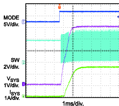
Mode On, Boost Mode V_{SYS\_SET}=5V , V_{BATT}=3.7V , R_{SYS\_LOAD}=2\Omega
