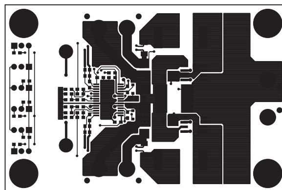
Copper Layer 1 Top
