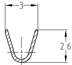
SECT. 断面 A-A
