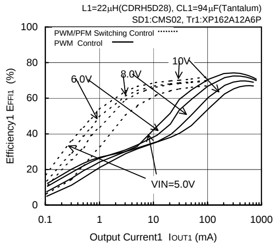
FOSC=300kHz, VOUT1=1.0V
