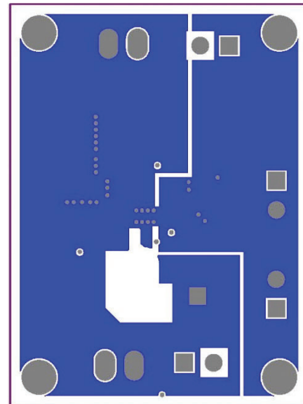
Fig. 26 - Bottom Layer
