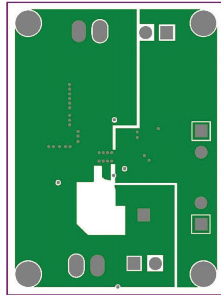
Fig. 25 - Inner Layer 1
