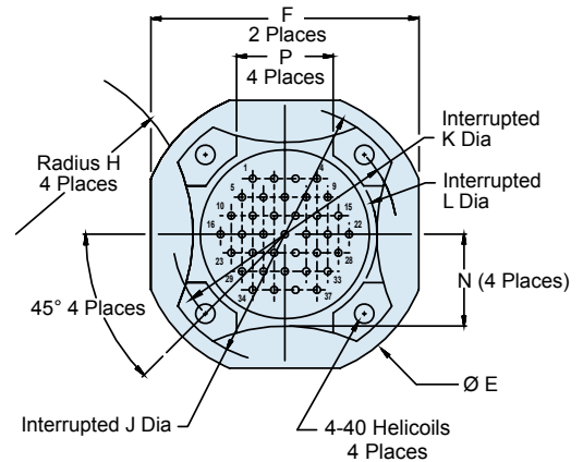
E - Dual Flange Jam Nut
