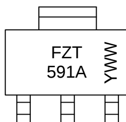
SOT223
