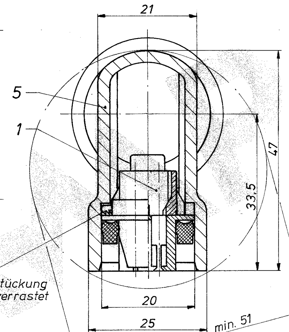
Schnitt A - B
