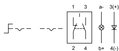
Wiring diagram 20
