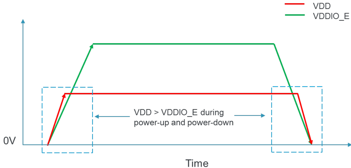
Figure 4. VDD &lt; VDDIO_E
