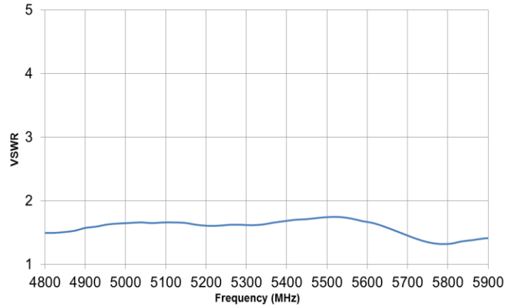
5 GHz VSWR
