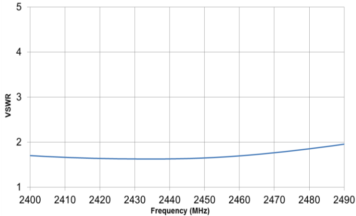
2.4 GHz VSWR
