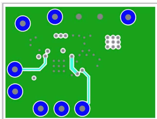
FIGURE 16. 3 rd LAYER
