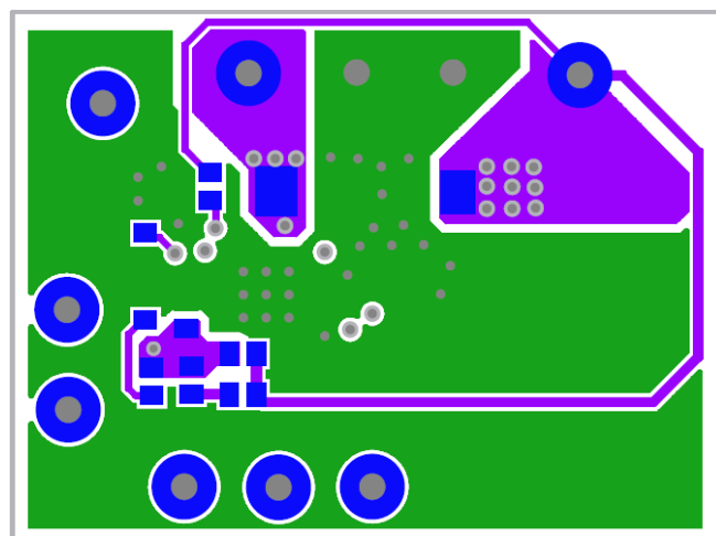
FIGURE 17. BOTTOM LAYER
