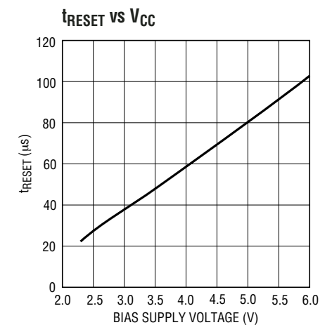
4213 G18
