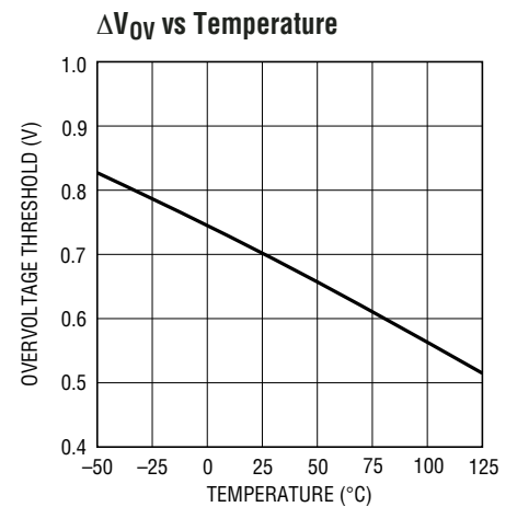
4213 G15
