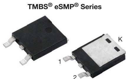
SlimDPAK (TO-252AE)
