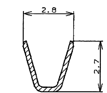
断面 "D" - "D" (SECT)
